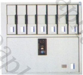
CAT 88-7D W880*D407*H880
